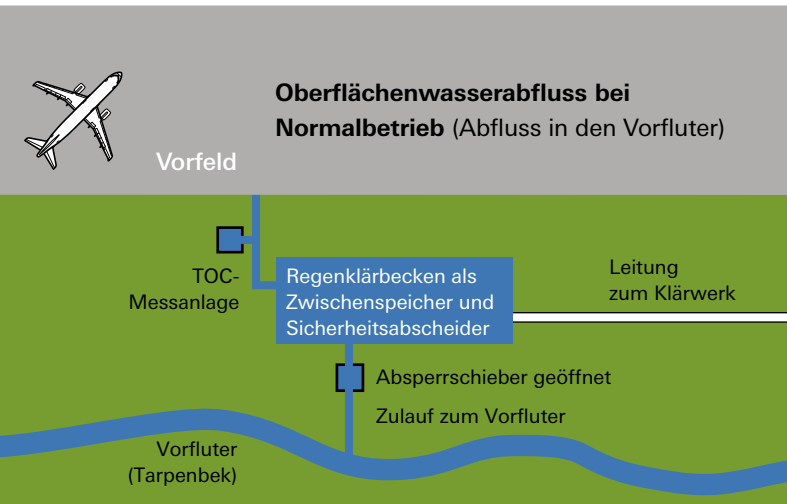
Funktionsprinzip der TOC-Anlage und des darüber gesteuerten Schiebersystems zum Schutz der Tarpenbek vor Enteisungsmitteln
